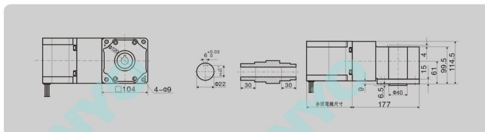
6GU-□RC(減速比5-500)
