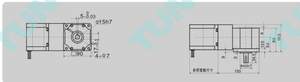
5GU-□RC(減速比5-500)
